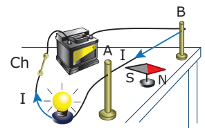
A bússola orienta-se na direção leste-oeste e fica ortogonal ao fio.
