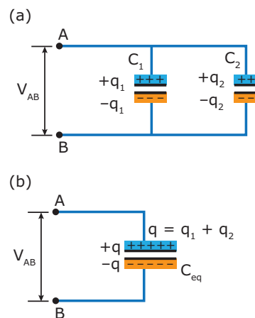
Figura 7: (a) Capacitores em paralelo; (b) capacitor equivalente.
