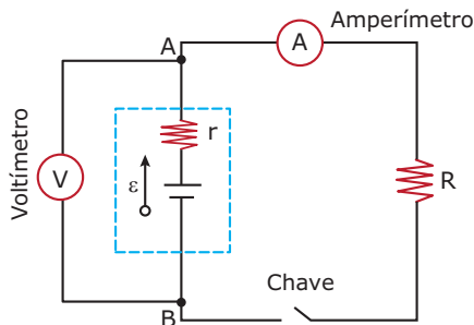
Figura 4: Montagem para determinar a f.e.m. e a resistência interna de uma fonte.
