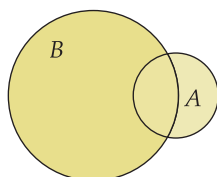
A \not\subset B
