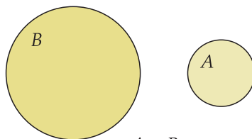
A \not\subset B
